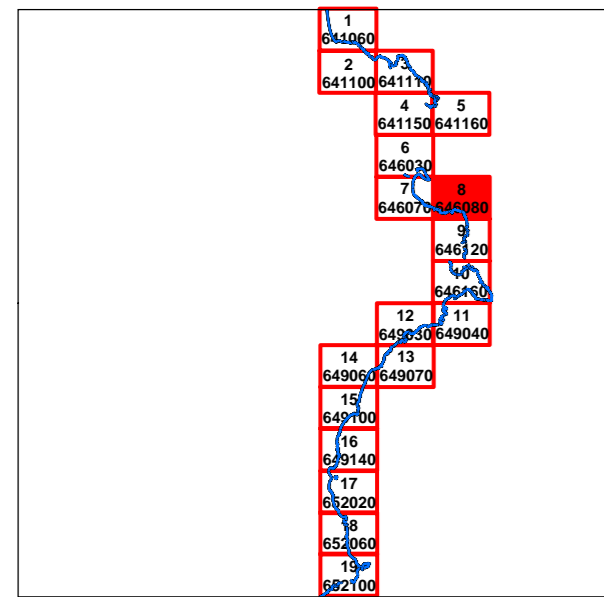
Carta delle opere marittime esistenti e in progetto N°8 Scala 1:5.000
